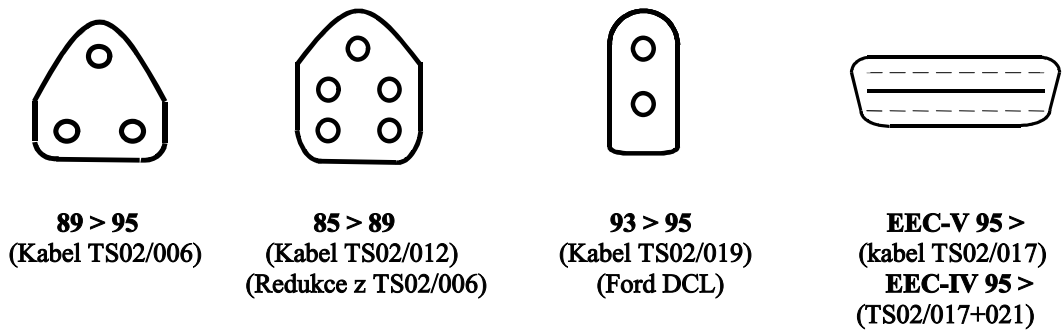
Vyobrazení zásuvek FORD
